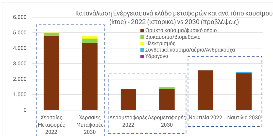
Σχήμα 6 Ενεργειακή κατανάλωση (σε 000 τιν) ανά κλάδο μεταφορών και τύπο καυσίμου, για τα έτη 2022 (ιστορικά) και το 2030 (προβλέψεις).
