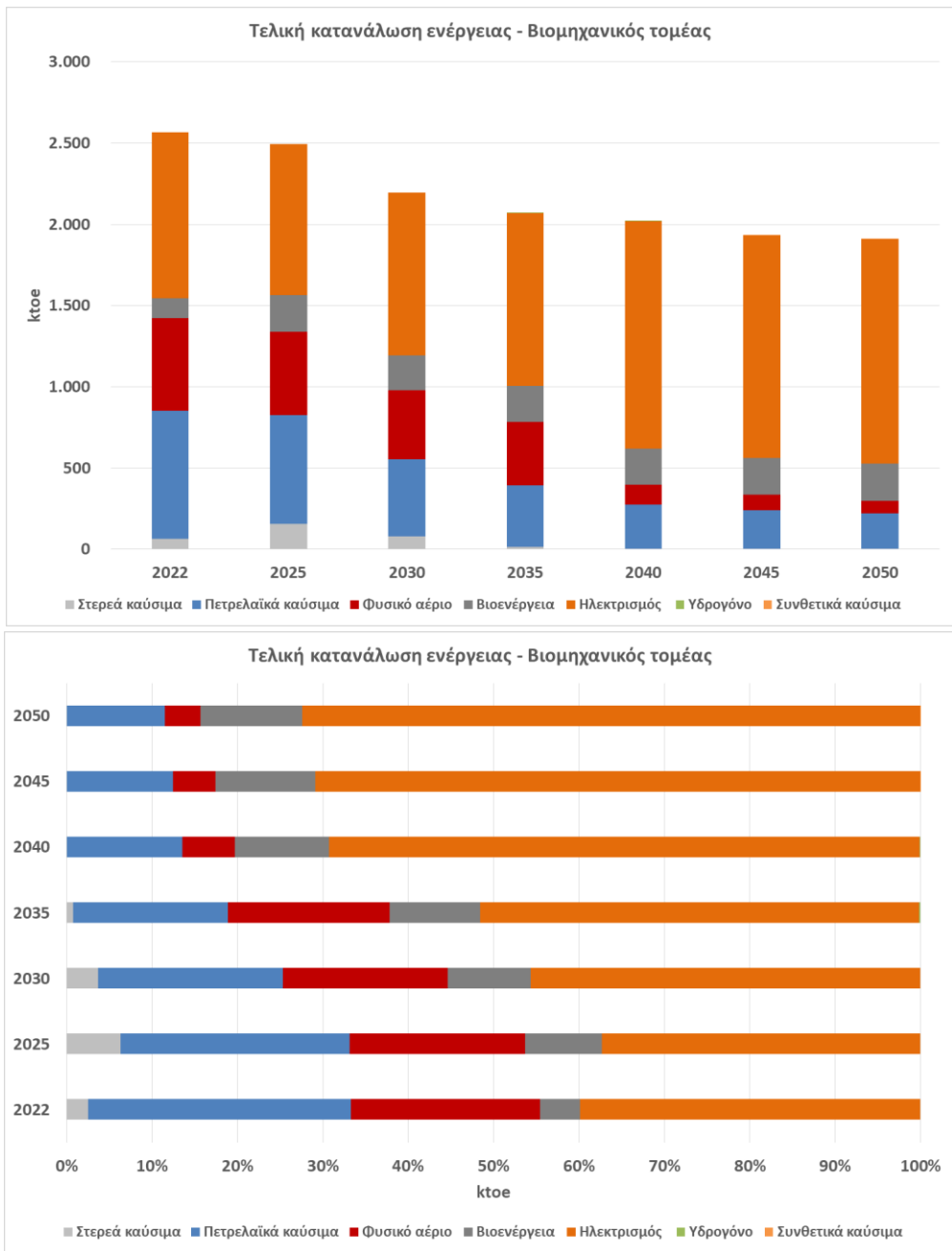
Σχήμα 56 Εξέλιξη τελικής κατανάλωσης ενέργειας στον τομέα της βιομηχανίας έως το έτος 2050.
