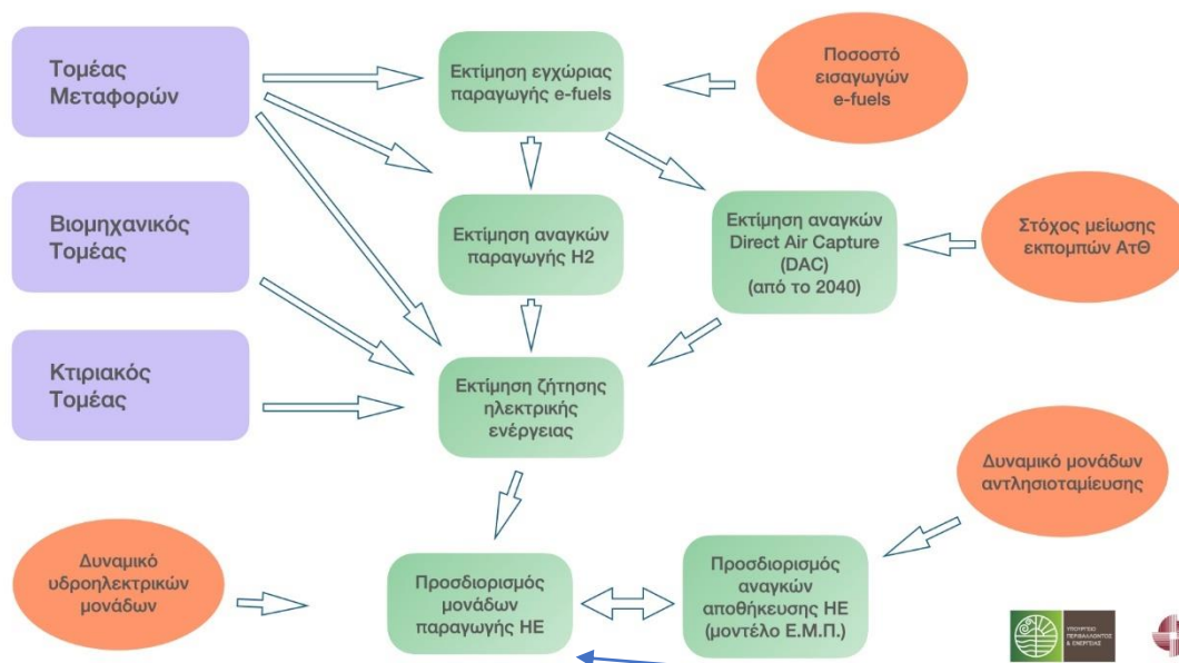
Σχήμα-Ε5 4 Σχηματική παρουσίαση ροής υπολογισμών προσδιορισμού μονάδων ηλεκτροπαραγωγής και αποθήκευσης ενέργειας.
