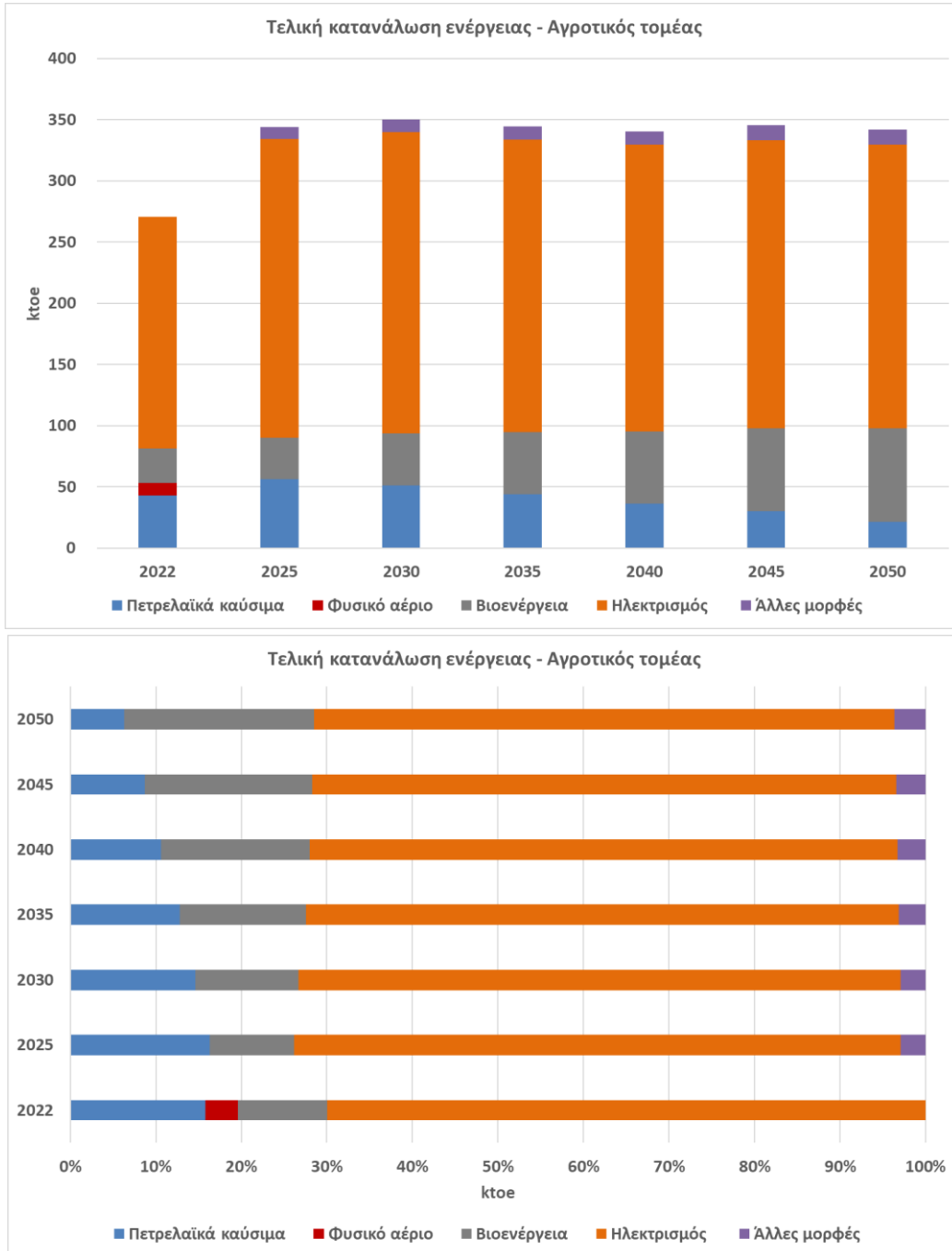
Σχήμα 57 Εξέλιξη τελικής κατανάλωσης ενέργειας στον αγροτικό τομέα έως το έτος 2050.
