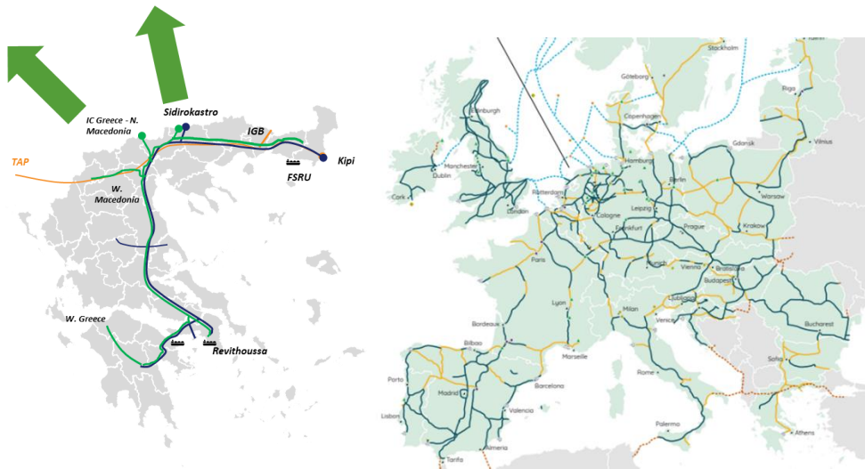
Εικόνα 3 Προγραμματισμένα δίκτυα μεταφοράς υδρογόνου στην Ελλάδα και την Ευρώπη 37 .
