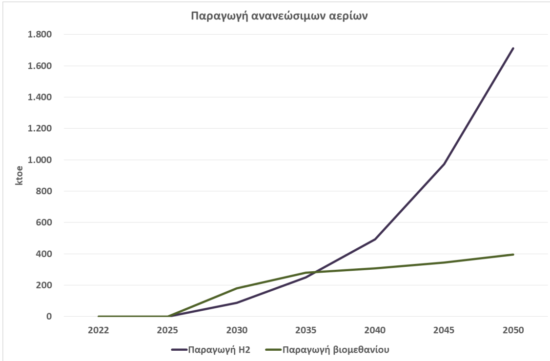
Σχήμα 34 Εξέλιξη παραγωγής ανανεώσιμων αερίων έως το έτος 2050.
