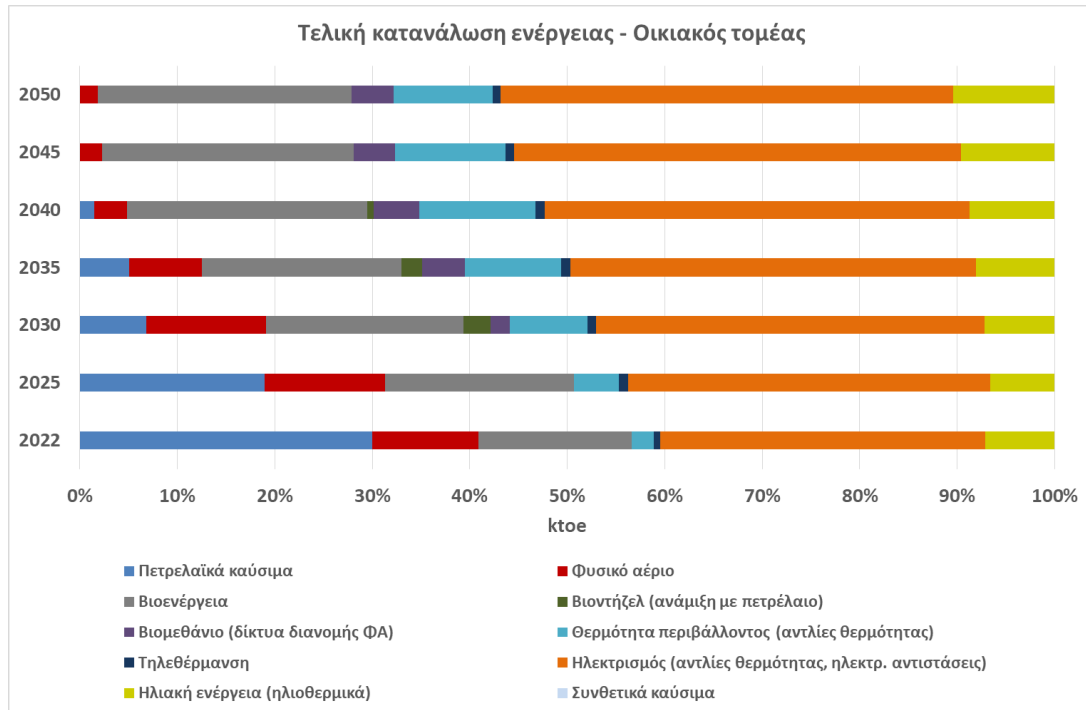
Σχήμα 45 Εξέλιξη τελικής κατανάλωσης ενέργειας στον οικιακό τομέα έως το έτος 2050.
